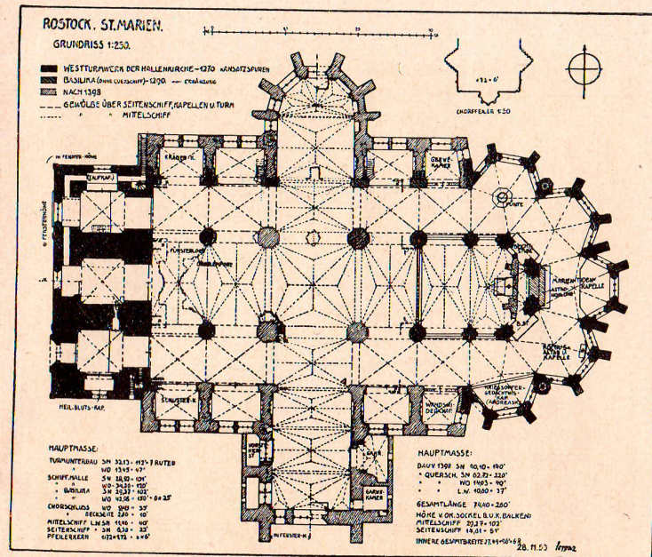
Grundriß von Lorenz 1953
